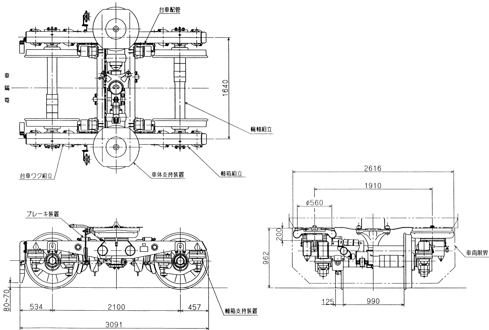
図 7-2 付随台車 (ND 728 T) 組立図
