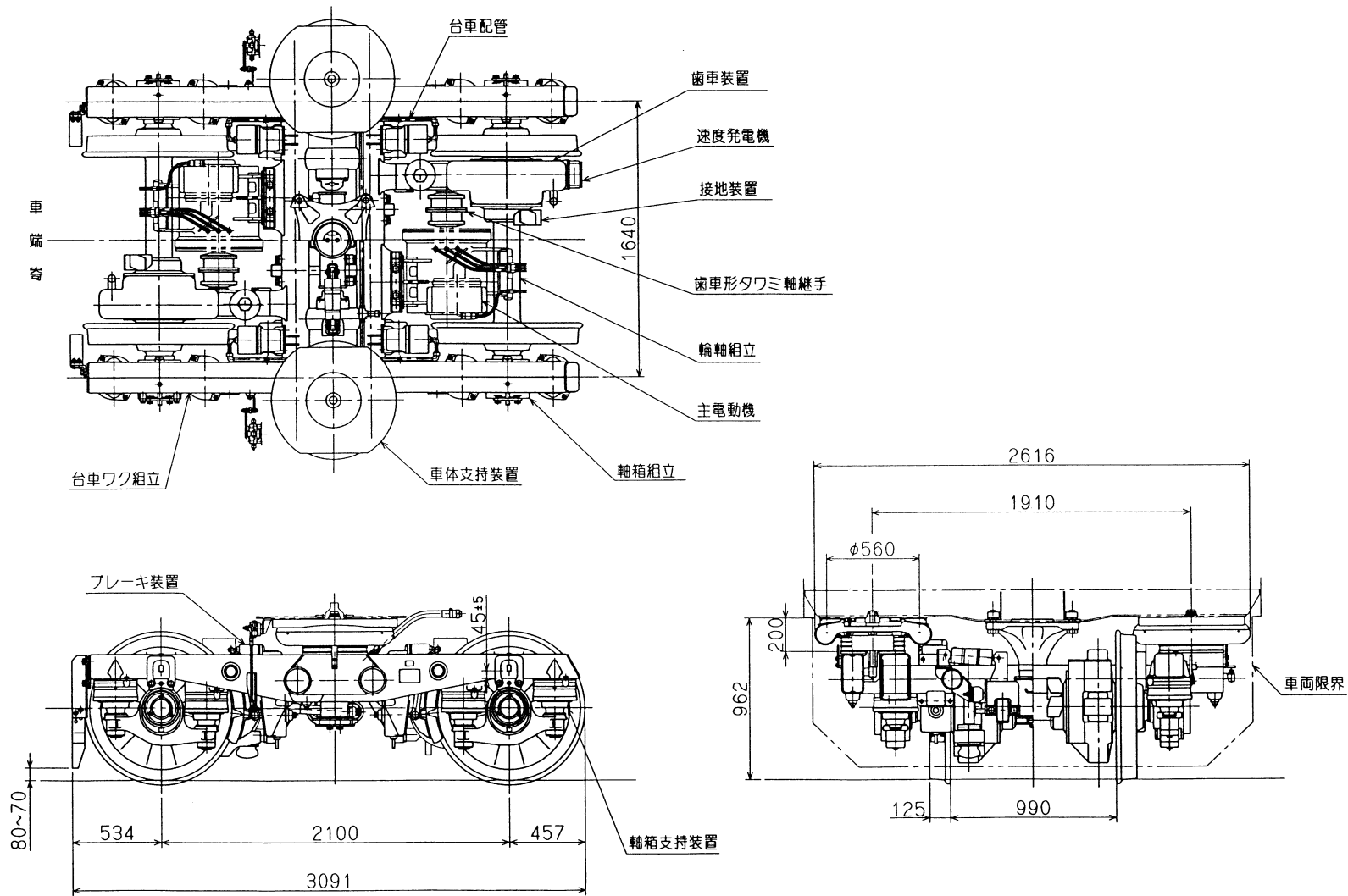
図7-1 電動台車 (ND 728) 組立図
