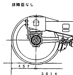
図9 台車組立図 (TR246D)
