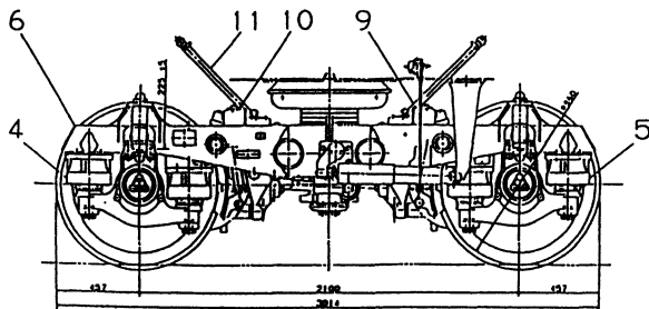
図12 DT56E組立図
