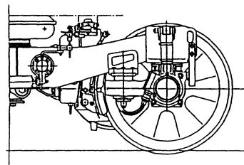
近鉄 22000系 図14 台車形式図 KD 304
