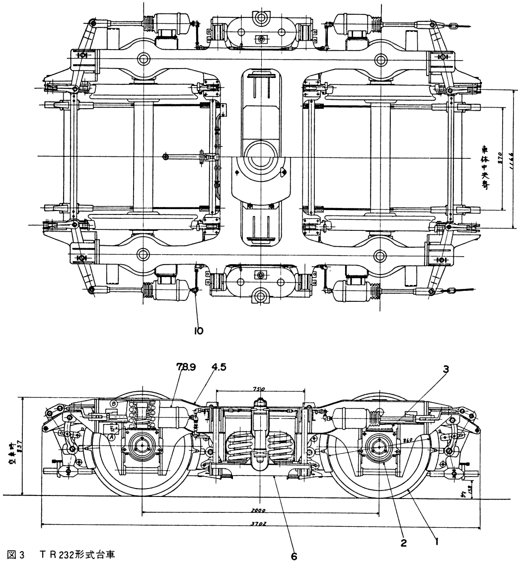
图 3 T R 232形式台車
