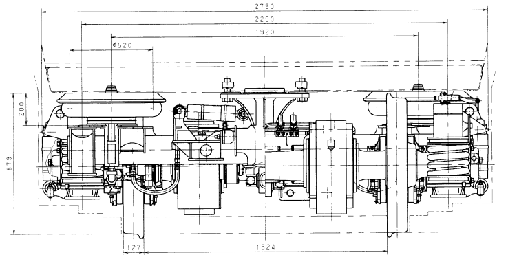
図6 電動台車組立 (TS-1024)
