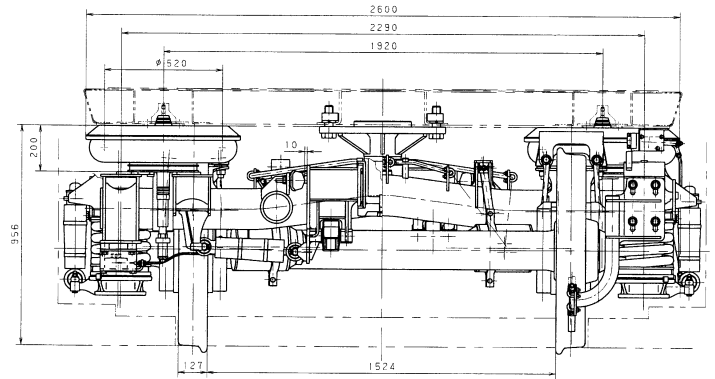
図6 付随台車組立 (TS-1023)
