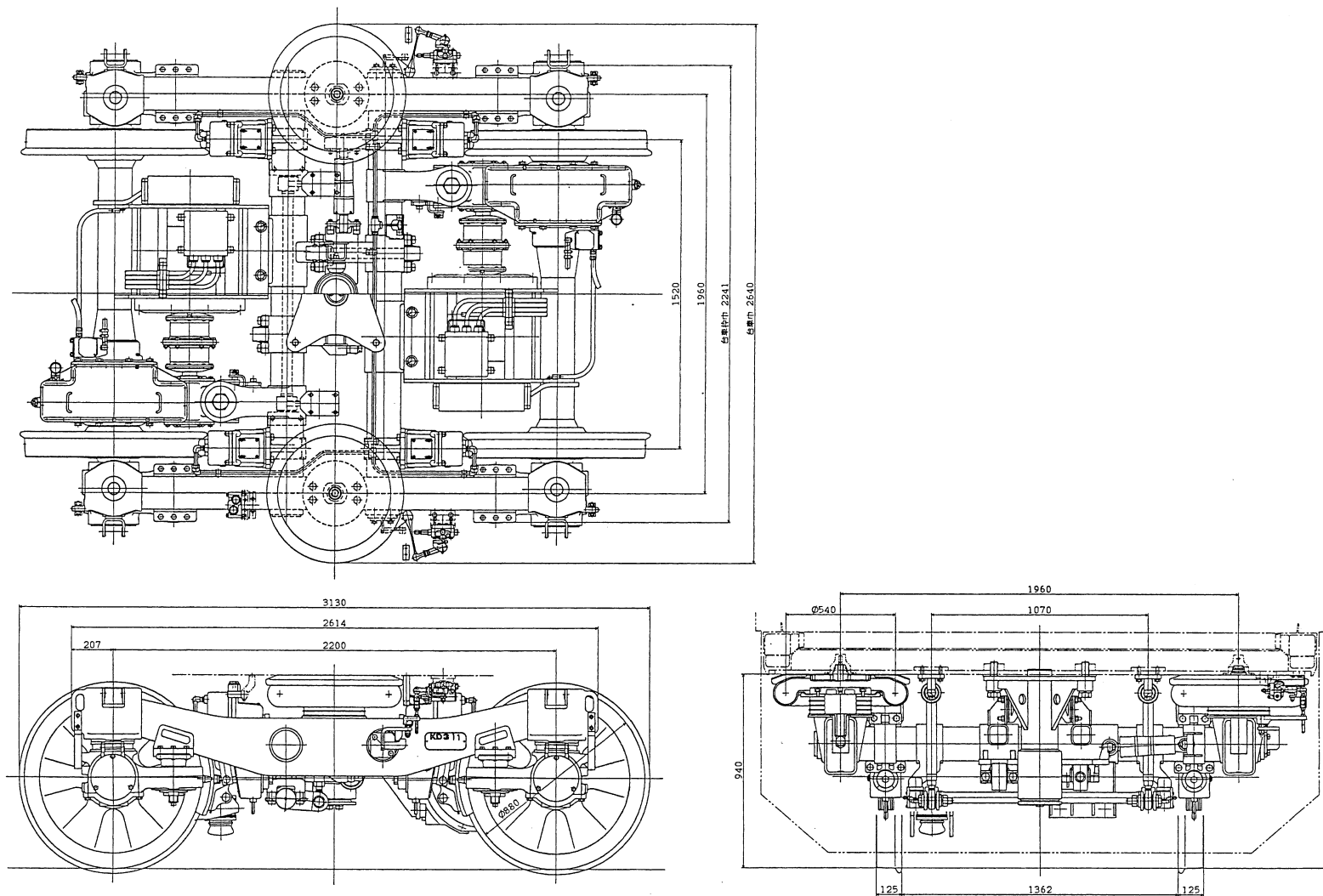
図17 台車組立 (KD311形)
