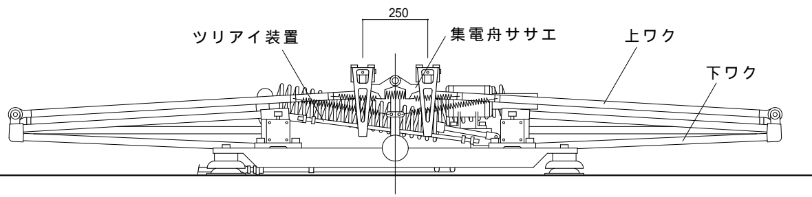
PS16型パンタグラフ
