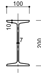
200 × 100 × 7 × 10 (26.0kg/m)
