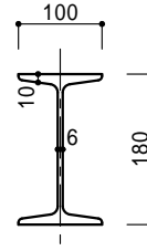
180 × 100 × 6 × 10 (23.6kg/m)
