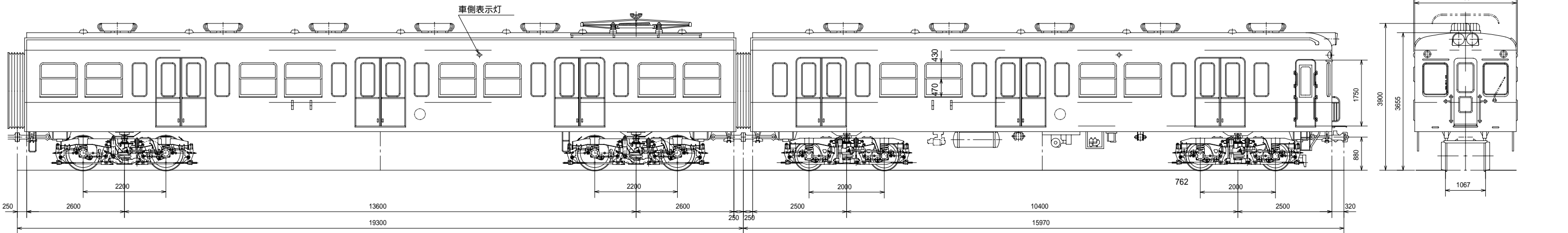
デハ2400形 M2
