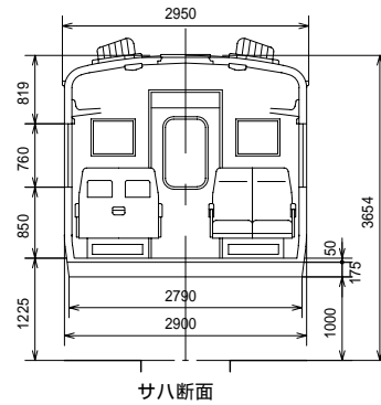
サハ断面
